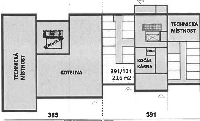
1.NP
